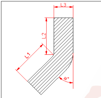
WIRBALIT® L Profil 5867
