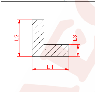
WIRBALIT® B Profil 2090/25x25x8
