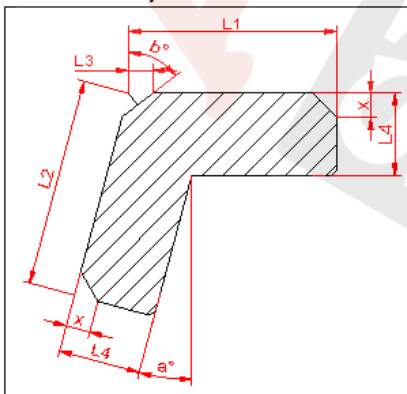
WIRBALIT® B/NIB Profil 5016
