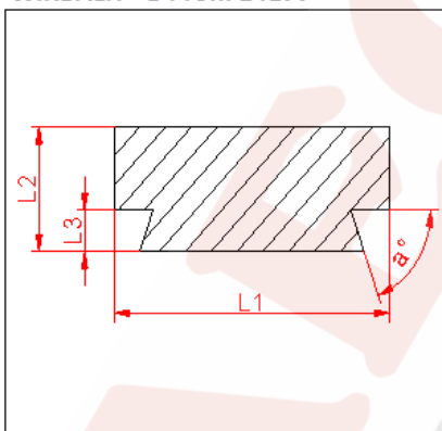
WIRBALIT® B Profil 14177
