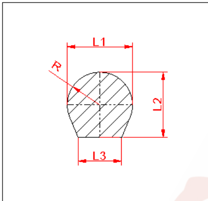
WIRBALIT® N Profil 2357
