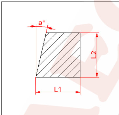
WIRBALIT® B Profil 5962
