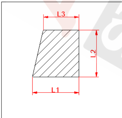
WIRBALIT® B Profil 2669
