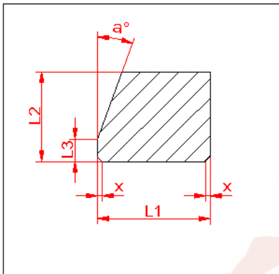
WIRBALIT® B Profil 13946
