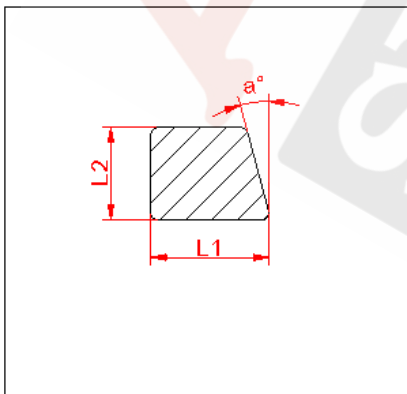
WIRBALIT® N Profil 5930
