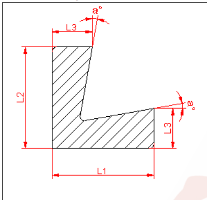
WIRBALIT® B/NIB Profil 5017
