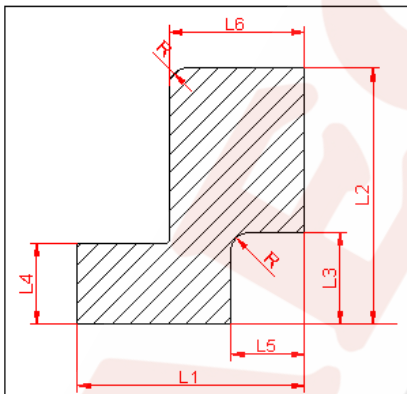
WIRBALIT® N Profil 2248
